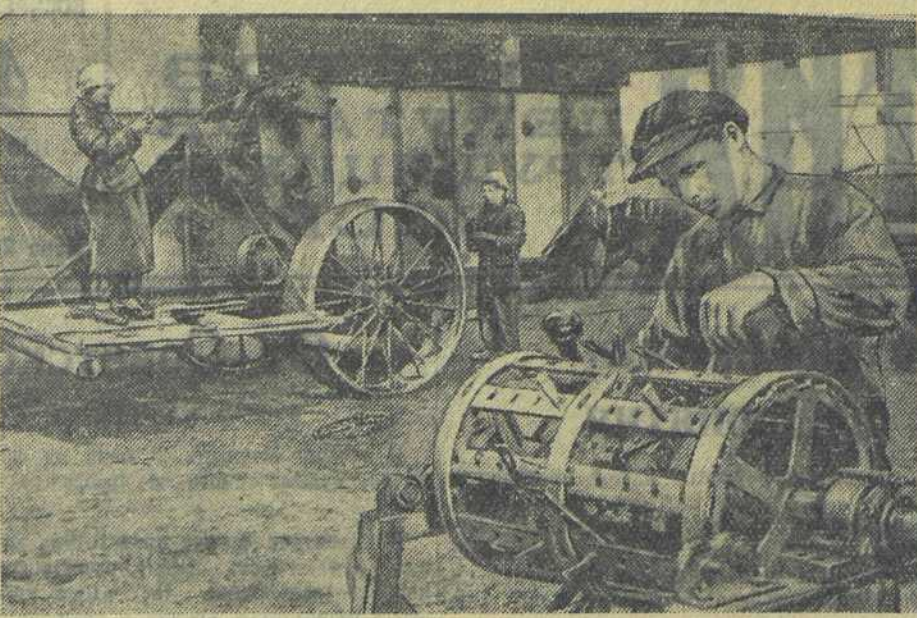
ПОДГОТОВКА К УБОРКЕ УРОЖАЯ. В Ершовской МТС Хабаровского края идёт ремонт комбайнов. На снимке: комбайнер М. И. Остапов производит сборку молотильного аппарата. Фото К. Фарафопова. (ТАСС).
